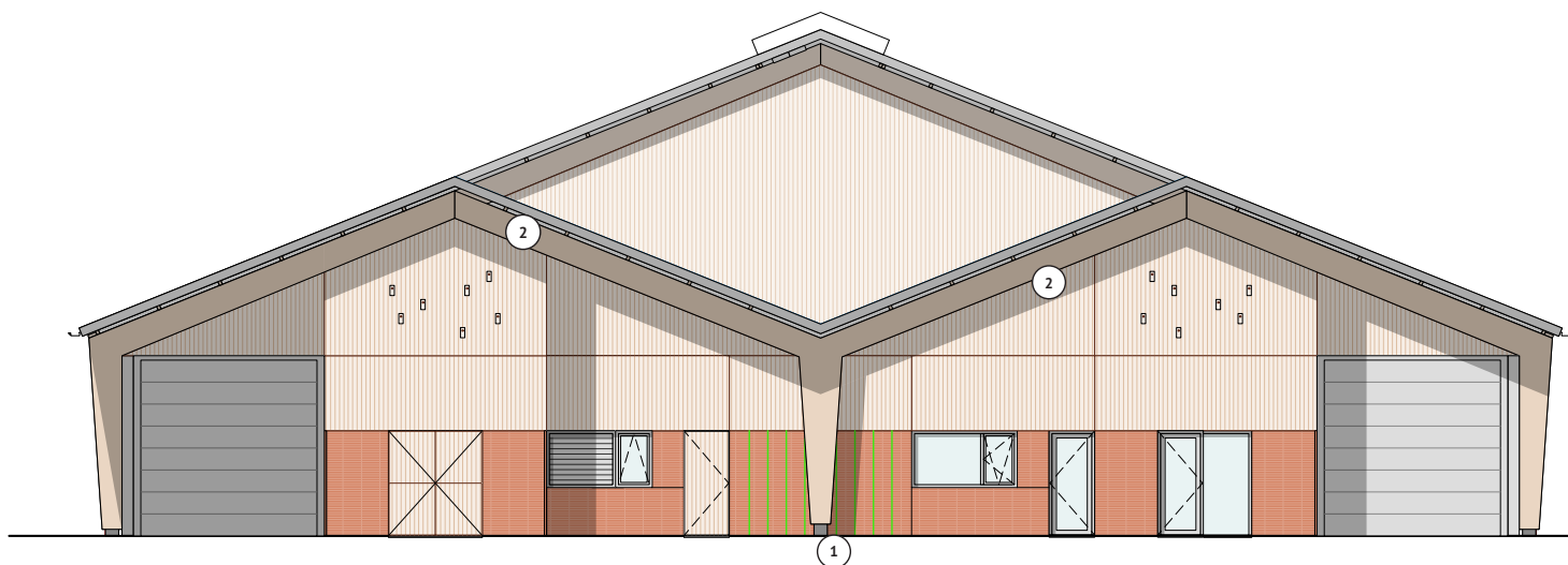
Voorgevel melkveeschuur
