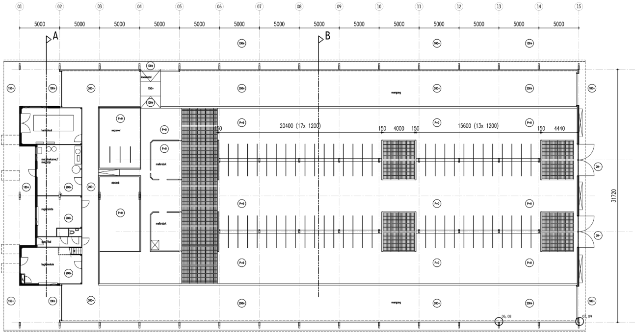
plattegrond
