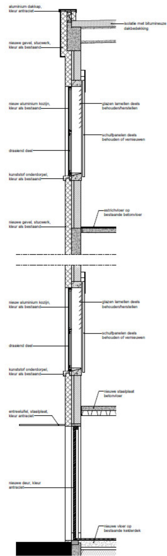
doorsnede nieuw
