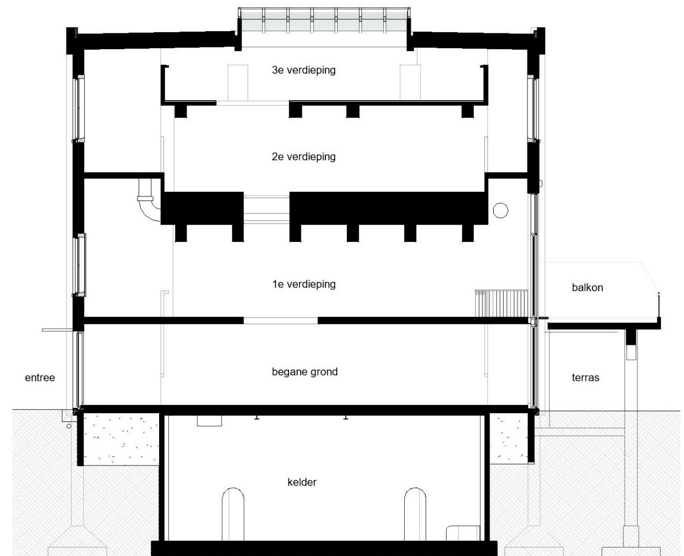
DOORSNEDE NIEUW
