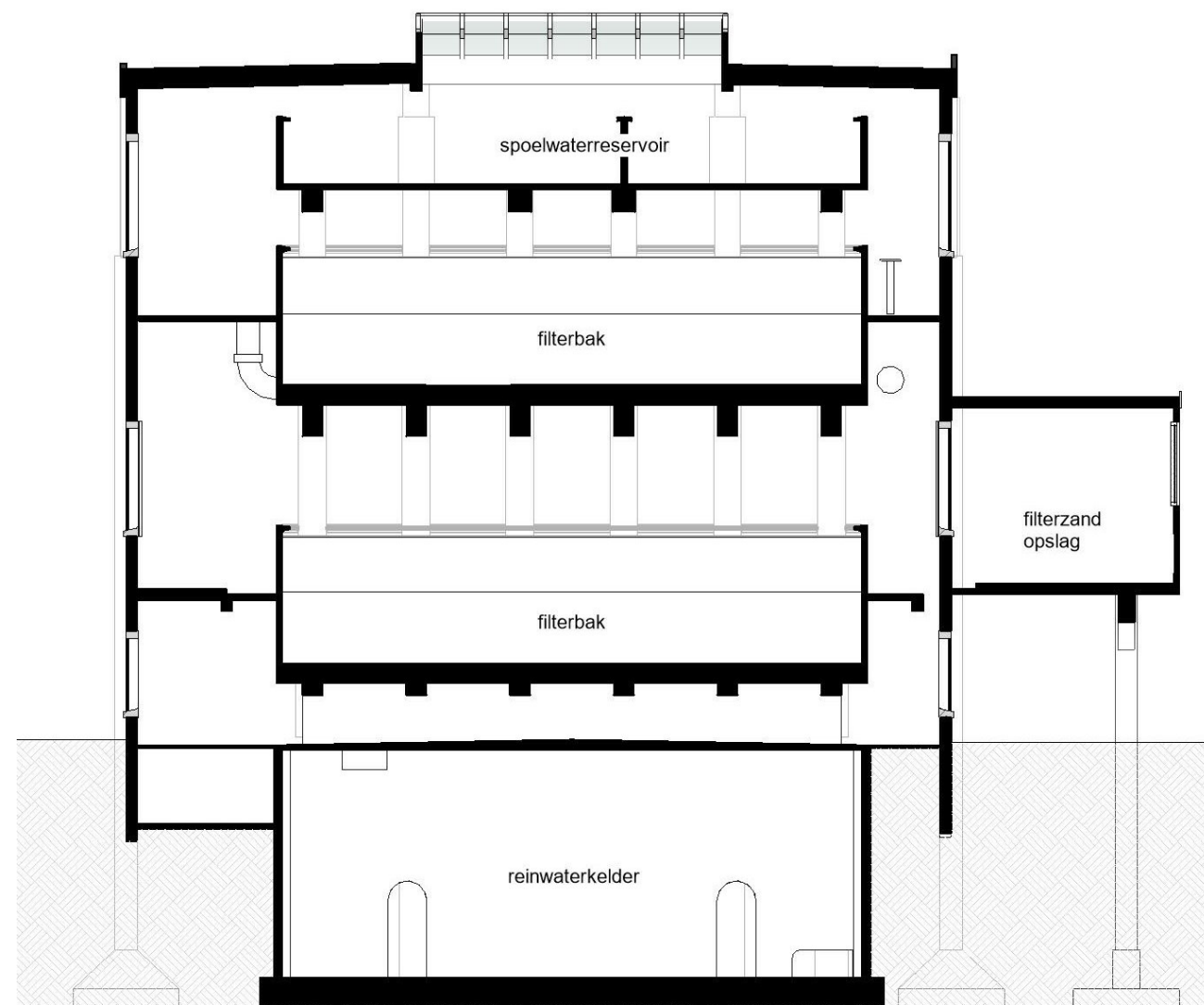
DOORSNEDE BESTAAND
